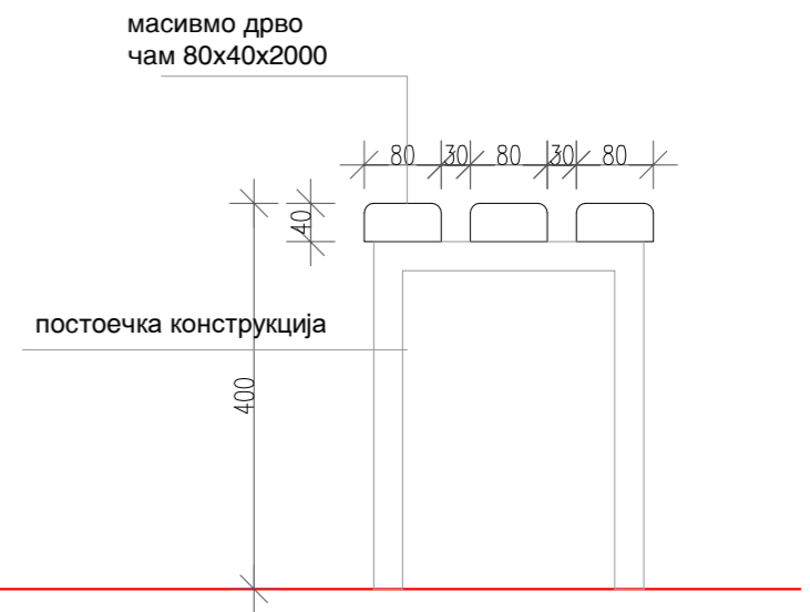
ПРЕСЕК 1-1
